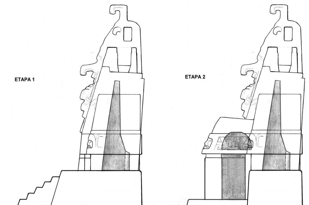
Figura 9 Corte hipotético norte sur, mostrando las dos principales etapas constructivas.
