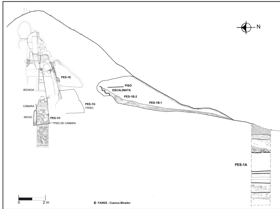
Figura 6 Corte norte sur de excavación en Estructura 1, Plaza A, El Pesquero (H. Iwamoto, H. Mejía, A. Portillo)
